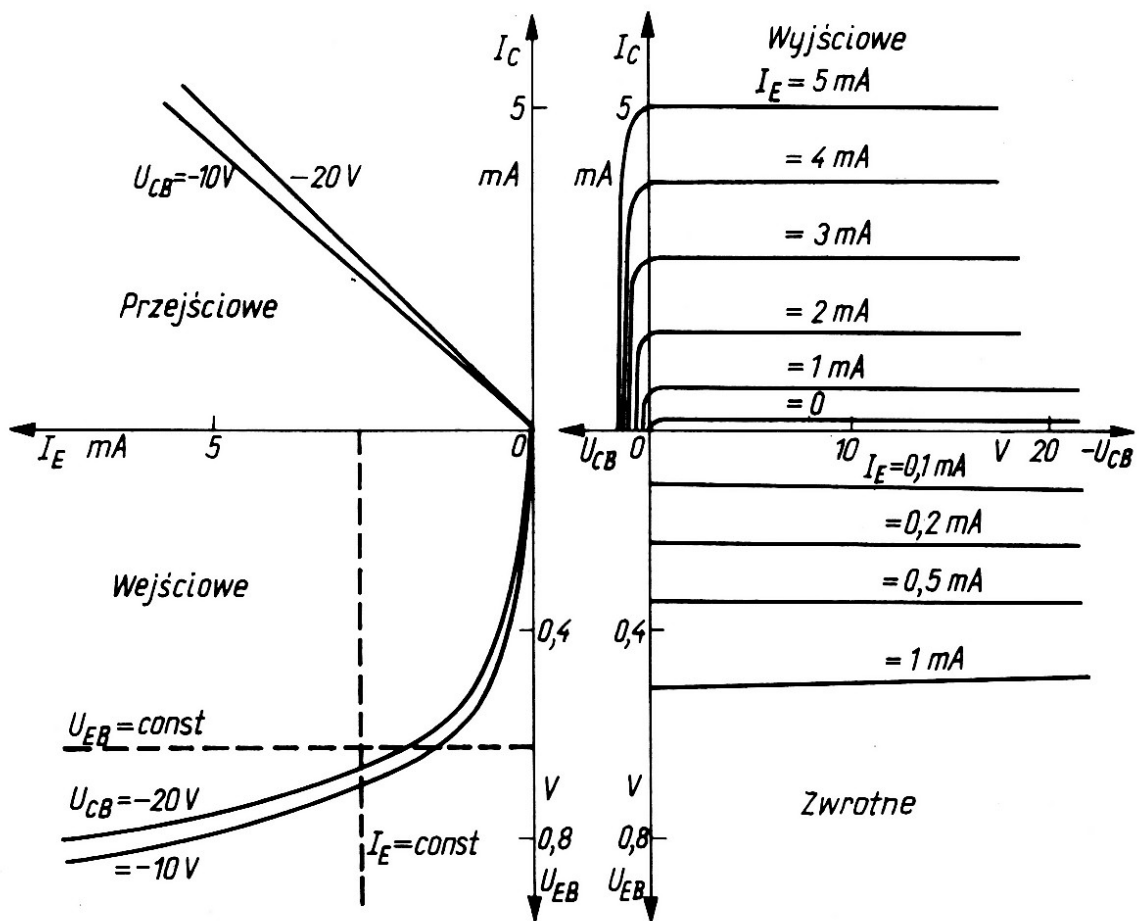
Charakterystyki statyczne tranzystora w układzie OB
