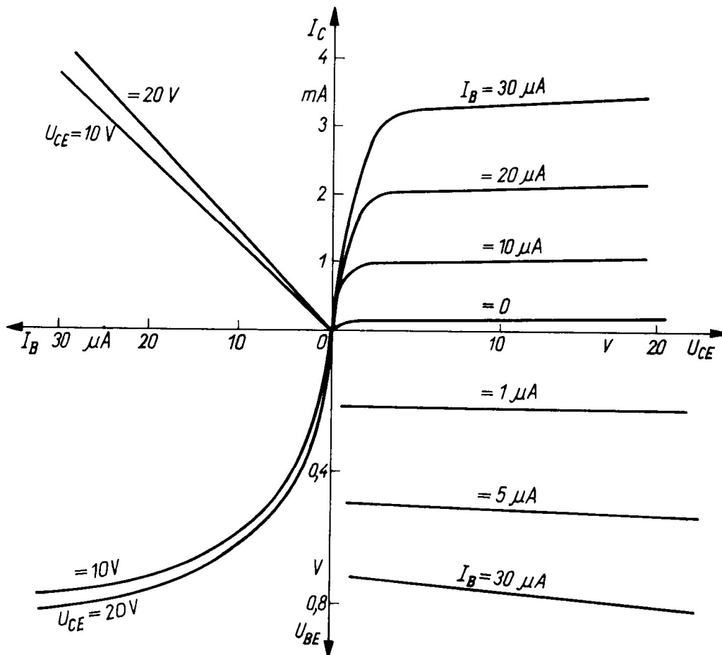
Charakterystyki statyczne tranzystora w układzie OE
